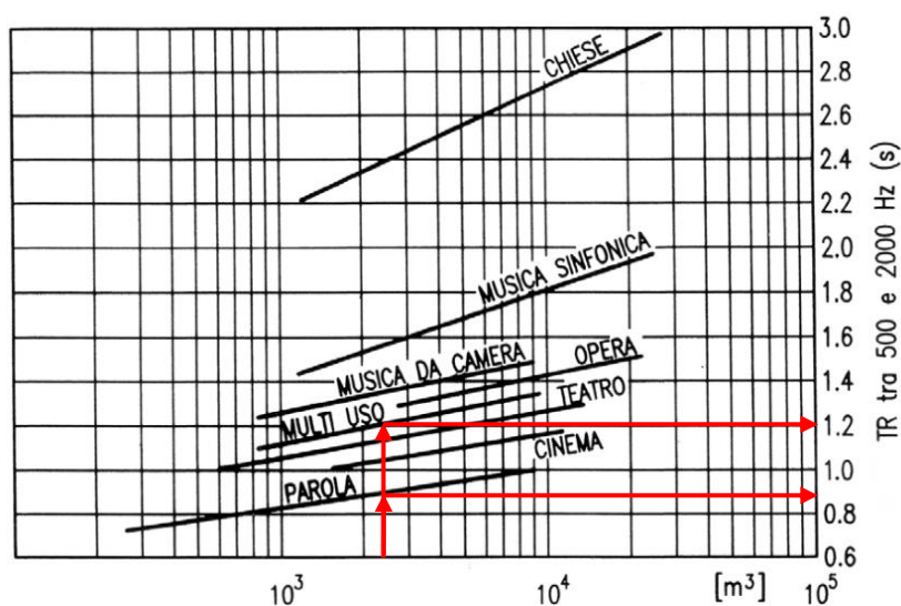
Figura 3 – Tempo di riverberazione ottimale in funzione del volume della sala
