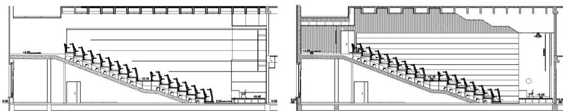
Figura 5 – Sezione della sala – stato di progetto ante studio acustico e stato di fatto
