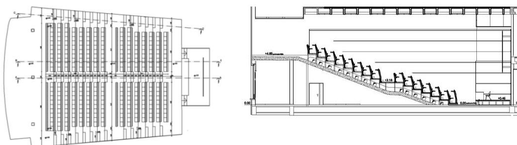
Figura 2 – Pianta e sezione della sala – stato di progetto
