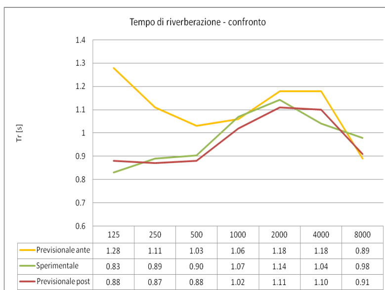
Figura 7 – Tempo di riverberazione – confronto
