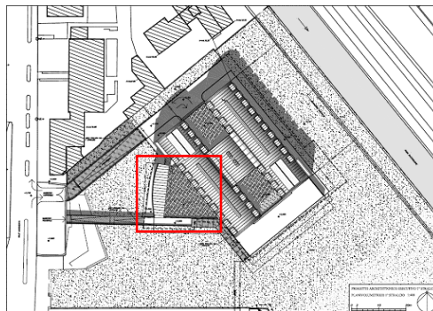
Figura 1 – Planimetria generale - I stralcio
